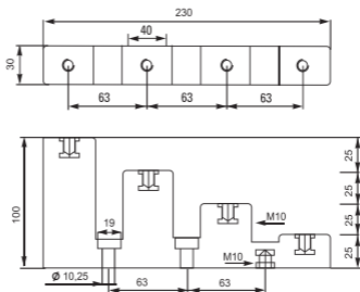
Изолятор «Лесенка» 900А 18кВ
