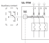
Fig. 1 - Wiring diagram
