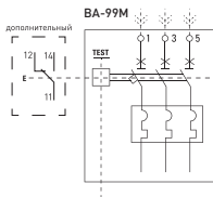
Рис. 1 - Принципиальная схема подключения дополнительного контакта
