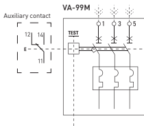
Fig. 1 - Wiring diagram
