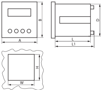
Рис. 2 Габаритные размеры
