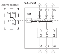
Fig. 1 - Wiring diagram
