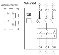
Fig. 1 - Wiring diagram
