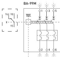
Рис. 1 - Принципиальная схема подключения аварийного контакта
