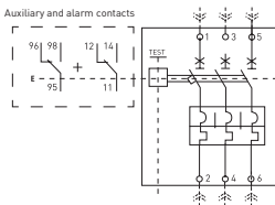
Fig. 1 - Wiring diagram
