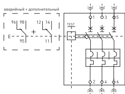
Рис. 1 - Принципиальная схема подключения дополнительного устройства
