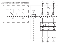
Fig. 1 - Wiring diagram
