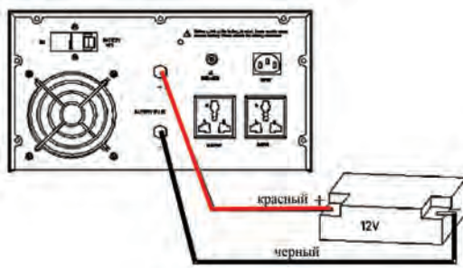
Схема подключения аккумуляторных батарей U=12V . Модель PSW-H PROxima 300 Вт – 1000 Вт
