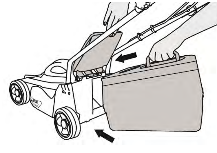
Рис. 3. Установка травосборника
