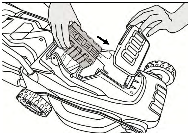
Рис. 4. Установка аккумуляторных батарей
