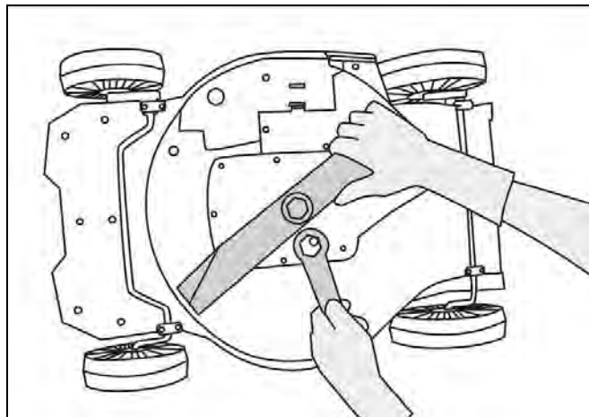
Рис.9. Замена лезвия
