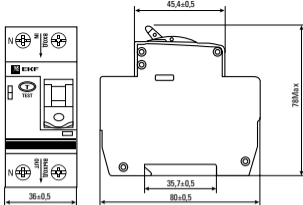
Рис.1 – Габаритные и установочные размеры УЗДП с номинальным рабочим током 10-63 А
