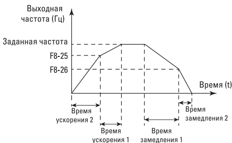
Рис. 6-19. Схема переключения времени ускорения/замедления
