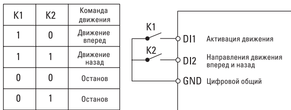
Рис. 6-7. Двухпроводной режим 2
