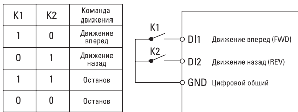
Рис. 6-6. Двухпроводной режим 1
