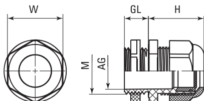
Рисунок 1. Основные размеры сальников.
