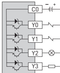
Выходы: NPN-транзисторы
