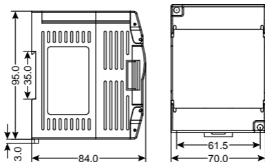
Рис. 1 – Габаритные размеры модулей REMF-D-16X, REMF-D-16Y-R, REMF-D-16Y-N, REMF-D-8X8Y-R, REMF-D-8X8Y-N, REMF-A-4Al, REMF-A-4A0, REMF-T-4TR, REMF-T-4TC
