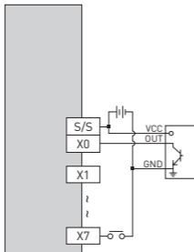
Входы: NPN-транзисторы
