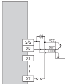
Входы: PNP-транзисторы
