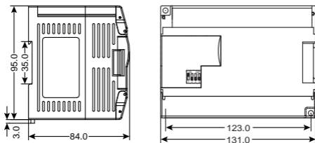
Рис. 2 – Габаритные размеры модулей REMF-D-40X, REMF-D-36Y-R, REMF-D-36Y-N
