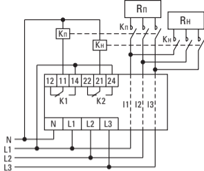
Рис. 2 Схема подключения
