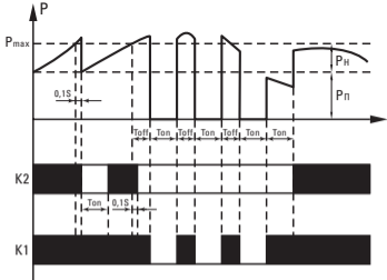
Рис. 1 Диаграмма работы ограничителя с приоритетной нагрузкой.
