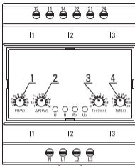
Рис. 3 Органы управления и индикации
