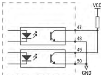
Рис. 6 Импульсные выходы
