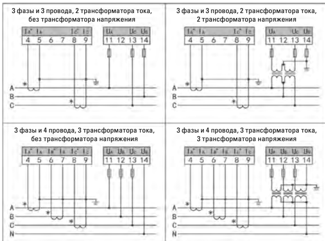
Рис. 5 Схема подключения
