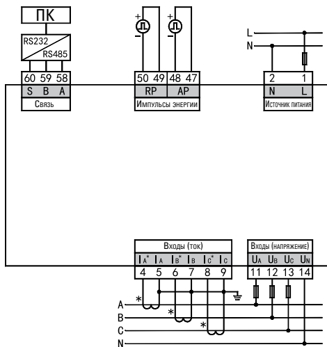
Рис. 4 Расположение клемм
