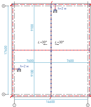
План отм. 0.000
