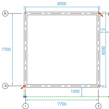
План отм. 0.000
