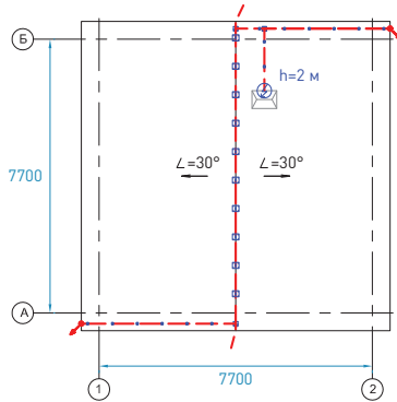
План кровли
