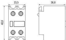
Рис. 1 Габаритные размеры ПКЗ-11, ПКЗ-20, ПКЗ-02
