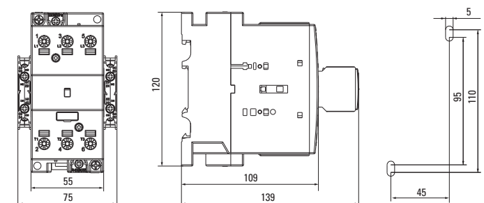
Рис. 6 – Габаритные и установочные размеры контакторов KM3 50A, KM3 60A, KM3 65A
