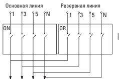
Схема соединения 4-х полюсного АВР
