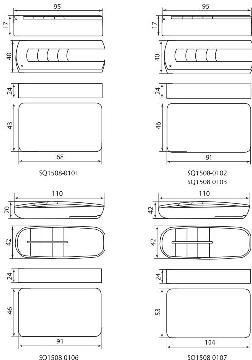
Рисунок 2. Габаритные размеры пультов и контроллеров, мм
