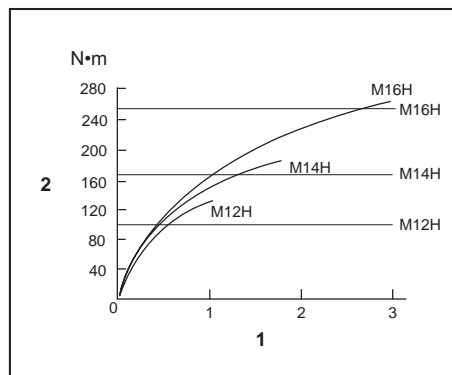
1. Festetid (sekunder) 2. Tiltrekkingmoment
