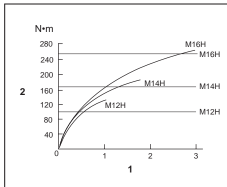
1. Åtdragnings-tid (sekunder) 2. Åtdragningsmoment
