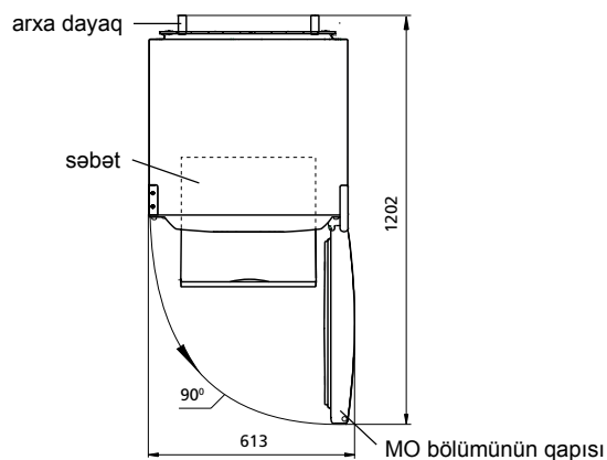
Resim 2 – Soyuducu (üstdən görünüşü)
