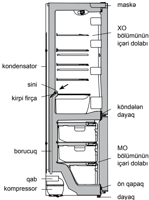
Resim 6 – XO bölümünün ərimiş axıntı sularının tökülmesi sxemi
