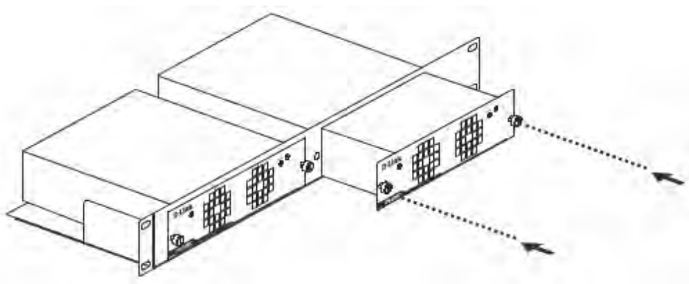
Рисунок 11 — Установка DPS-500A в DPS-800
