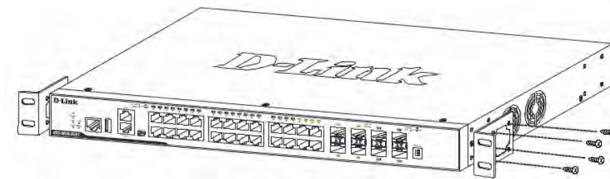
Рисунок 2 — Крепление кронштейнов
