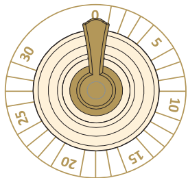
1 - Таймер (0-30 минут)
