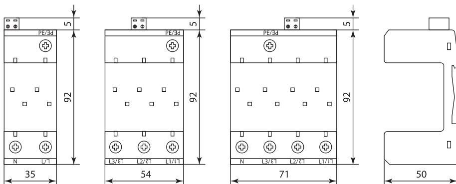
Рисунок 1. Габаритные размеры, мм
