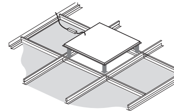
Рис. 1. Монтаж встраиваемого светильника в подвесной потолок типа «Армстронг»
