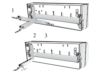
Формировать соединяющий провод.
