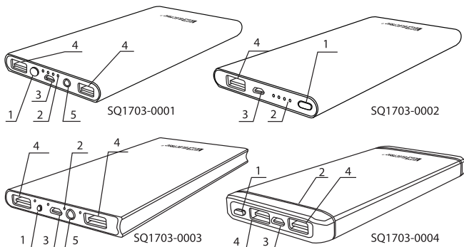
Рисунок 1. Конструкция аккумуляторов
