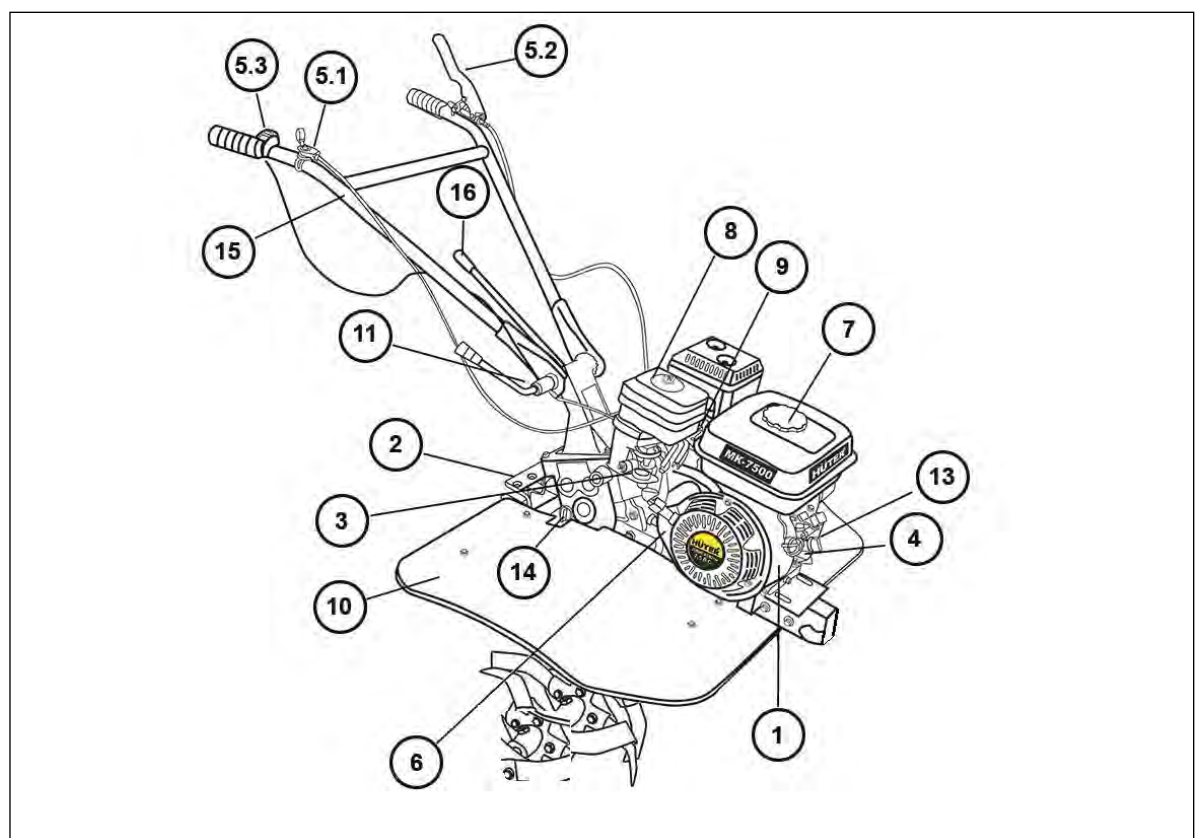
Рис. 2. Общий вид 2
