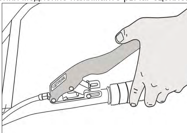
Рис. 36. Нажатие рычага сцепления
