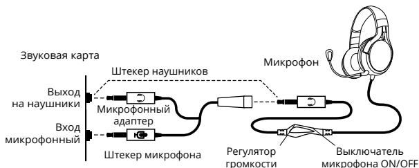
Рис. 2. Схема подключения
