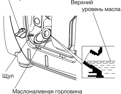
Маслоналивная горловина
