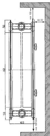
Схема установки радиатора
