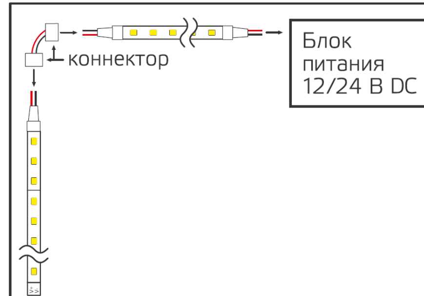
Рис. 1. Подключение коннектора
