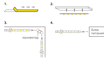
Рис. 3. Порядок монтажа
