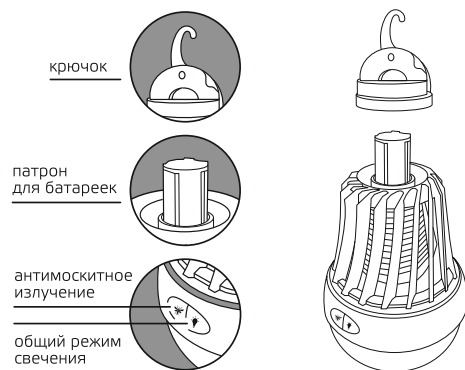
Рис.1. Схема антимоскитного светильника GMQ02
