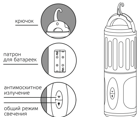
Рис.2. Схема антимоскитного светильника GMQ03
