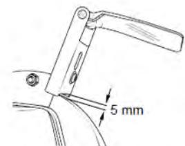
Рис. 4. Установка защитного экрана
