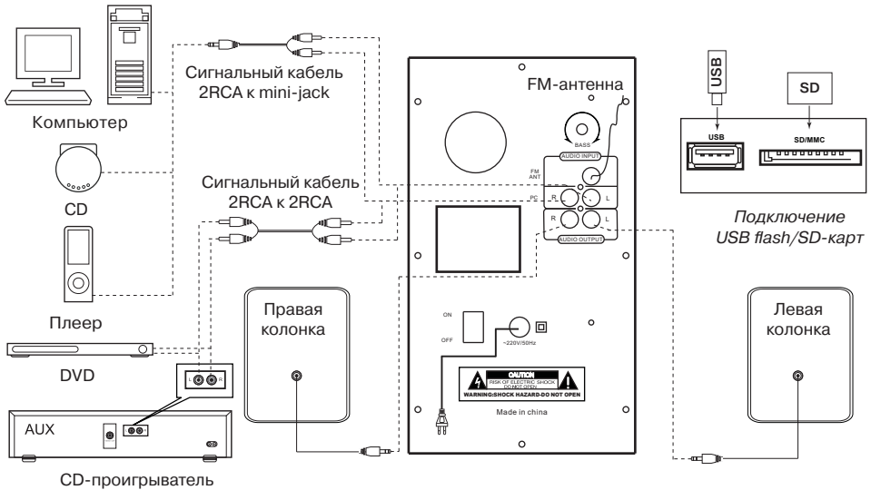
Рис. 4. Схема подключения
