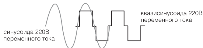
Сравнение квазисинусоиды и чистой синусоиды
