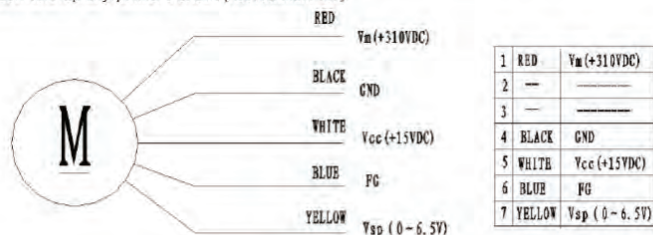
Вентилятор внутреннего блока (постоянный ток)
