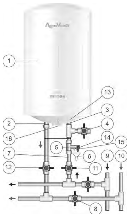
Рисунок 1. Схема подключения ЭВН к водопроводу
