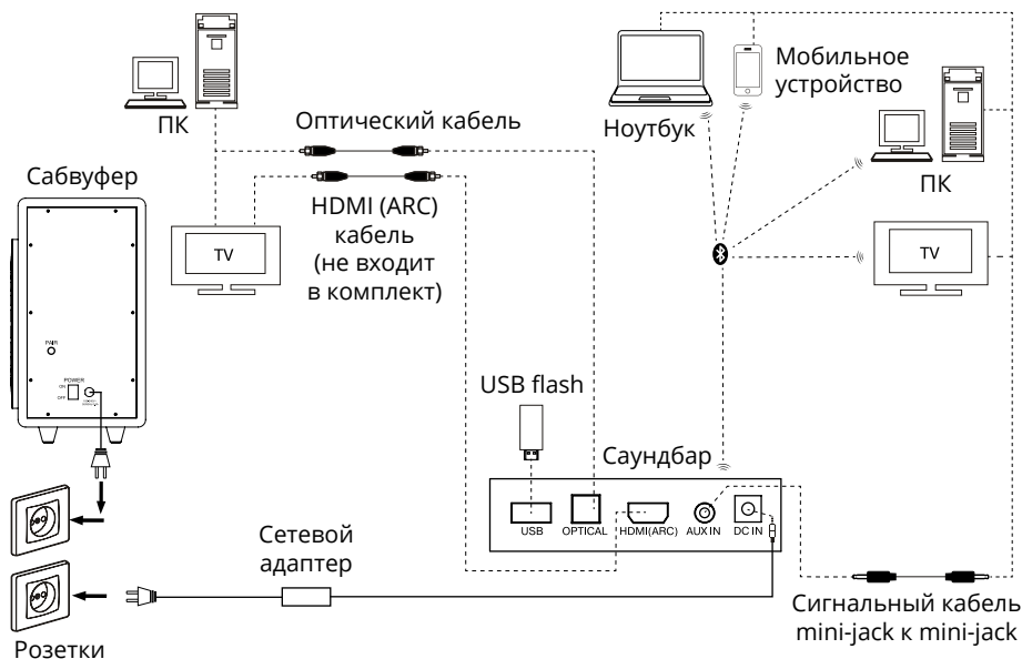
Рис. 4. Схема подключения
