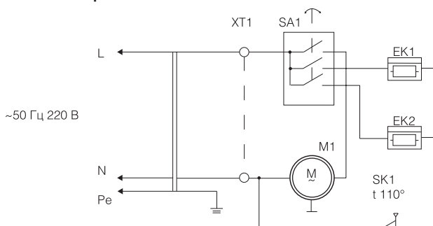
Схема комутации переключателя
