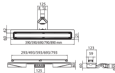
Боковой S-образный сифон D50-H60-42L/min
