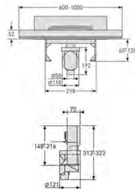
Вертикальный S - образный сифон D50/105мм-H30/80мм-48L/min
