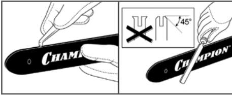
Рис. 33 Обслуживание шины
