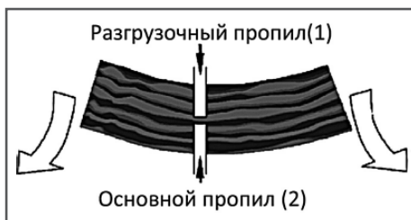
Рис. 17 Распиливание дерева, когда его нижняя часть находится под напряжением
