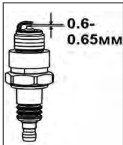
Рис.19 Свеча зажигания
