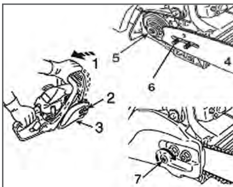
Рис. 2 Установка шины
