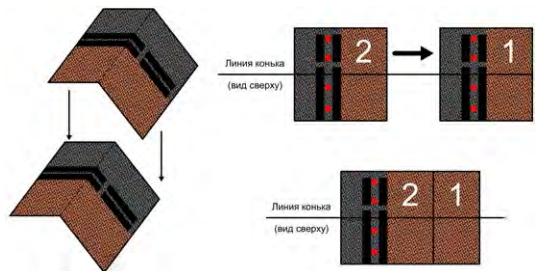
Рис. 31. Устройство рёбер скатов и коньков.
