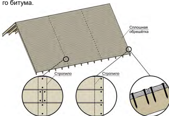
Рис. 6. Укладка сплошного основания из шпунтованной или обрезной доски.
